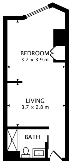
SUITE 404 40.3 m 2
